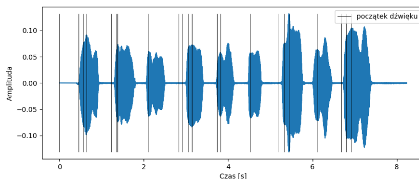
Rysunek 2.10: „Wlaził kotek na płótek v.2”, Surf method n_0 = 2500 , threshold = 0.01
