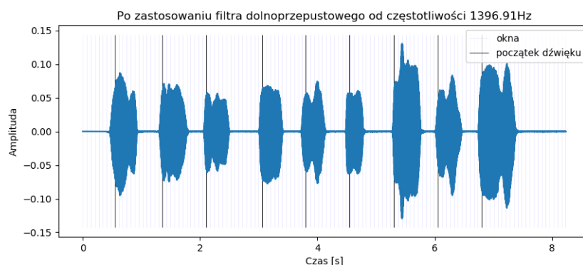
Rysunek 2.4: „Wlaził kotek na płótek v.2”, Magnitude method n_0 = 1500 , threshold = 0.015 , \epsilon = 6000
