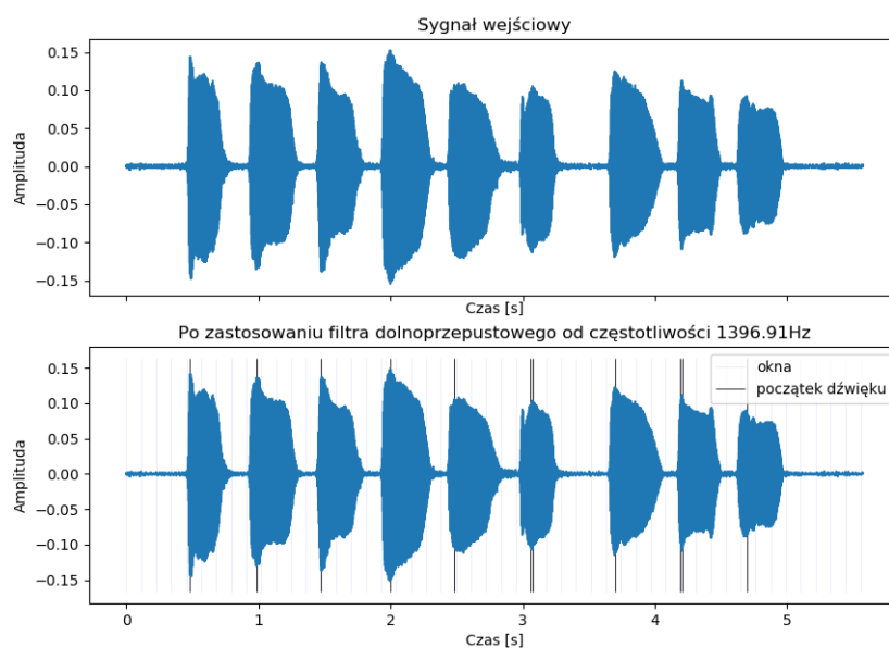
Rysunek 2.1: „Wlaził kotek na płotek v.1”, Magnitude method n_0 = 2500 , threshold = 0.006
