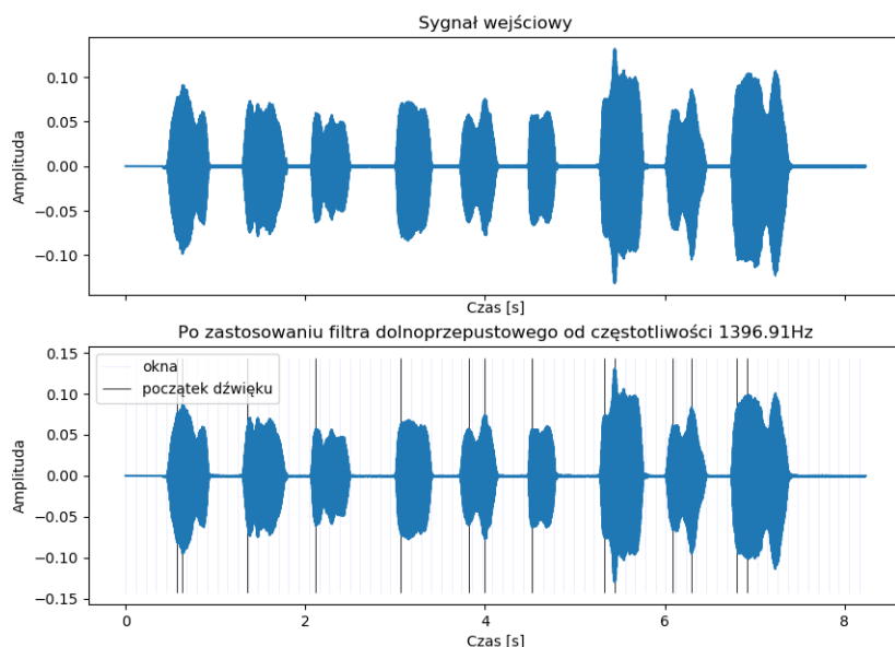
Rysunek 2.3: „Wlaził kotek na płotek v.2”, Magnitude method n_0 = 2500 , threshold = 0.015
